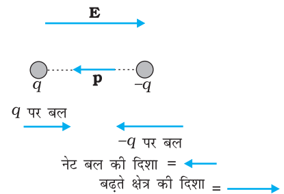
चित्र 1.20 द्विध्रुव पर वैद्युत बल (a) \mathbf{p} क्षेत्र \mathbf{E} के समांतर (b) \mathbf{p} क्षेत्र \mathbf{E} के प्रतिसमांतर।
