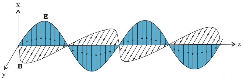
चित्र 8.3 एक रेखीय ध्रुवित वैद्युतचुंबकीय तरंग जो z -दिशा में गमन कर रही है और जिसका दोलनकारी विद्युत क्षेत्र \mathbf{E} , x -दिशा के अनुदिश एवं दोलनकारी चुंबकीय क्षेत्र \mathbf{B} , y -दिशा के अनुदिश है।
