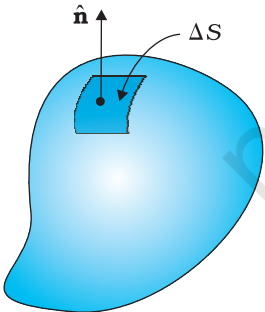
चित्र 1.16 अभिलंब \hat{\mathbf{n}} तथा \Delta \mathbf{S} को परिभाषित करने की परिपाटी।
