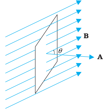
चित्र 6.4 एकसमान चुंबकीय क्षेत्र B में रखा पृष्ठ क्षेत्रफल A वाला एक समतल।
