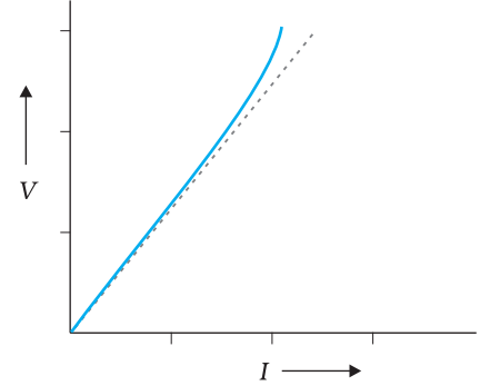
चित्र 3.5 बिंदुवित रेखा रैखिक ओम-नियम को निरूपित करती है। सतत रेखा अच्छे चालक के लिए V तथा I के संबंध को दर्शाती है।
