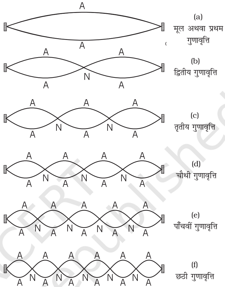
चित्र 14.13 दोनों सिरों पर परिबद्ध तानित डोरी में दोलन की प्रथम छः गुणावृत्तियाँ।
