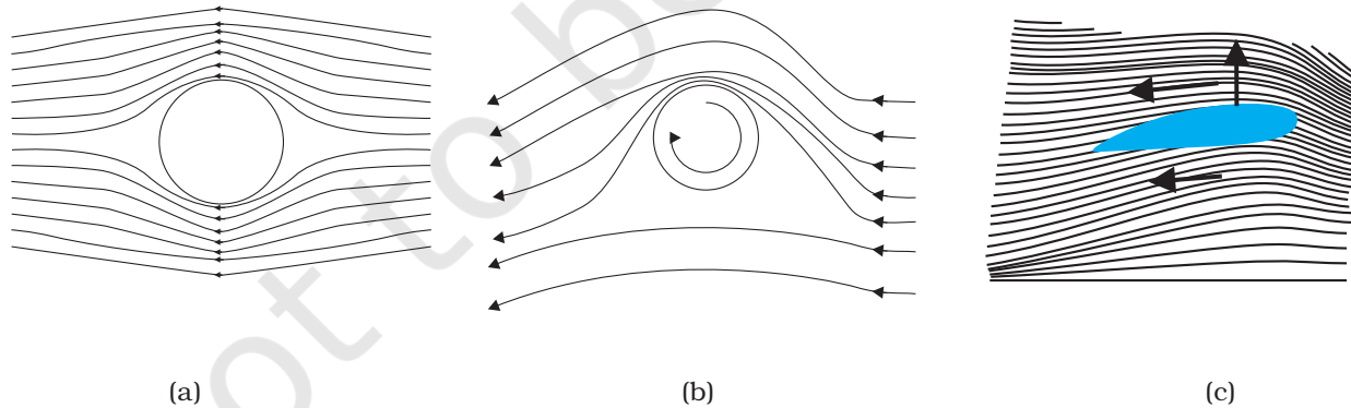
चित्र 9.11 (a) अधूर्ण गतिमान गोले के समीप तरल (b) एक घूमते गतिमान गोले के निकट से गुजरने वाले तरल का धाराप्रवाह (c) ऐयरोफॉयल के समीप से गुजरने वाली वायु में धारा रेखाएँ।
