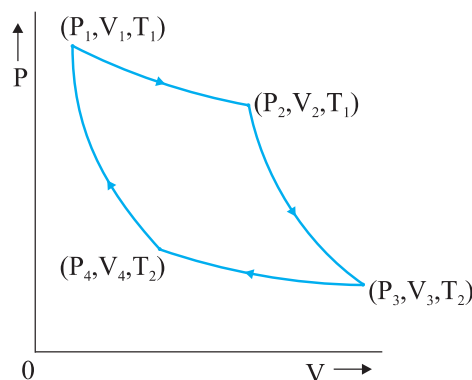
चित्र 11.9 किसी ऊष्मा इंजन के लिए कार्नों चक्र जिसमें कार्यकारी पदार्थ के रूप में आदर्श गैस का उपयोग होता है।
