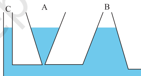
चित्र 9.4 द्रवस्थैतिक विरोधोक्ति की व्याख्या। तीन पात्रों A , B और C में समान ऊँचाई तक जल भरा है परन्तु सभी में जल का परिमाण भिन्न-भिन्न है।
