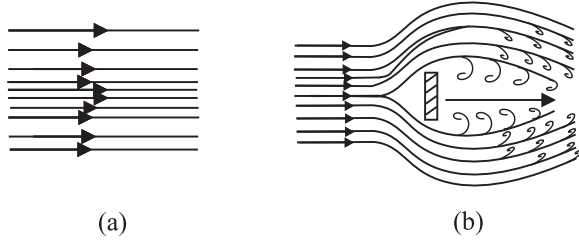
चित्र 9.8 (a) तरल प्रवाह की कुछ धारा रेखाएँ (b) प्रवाह के लंबवत् रखी चपटी प्लेट से टकराता वायु जेट। यह प्रक्षुब्ध प्रवाह का एक उदाहरण है।
