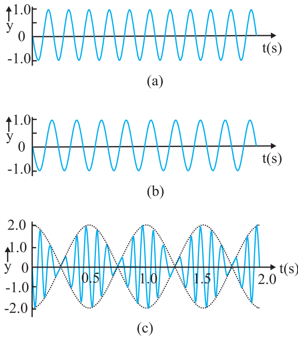
चित्र 14.16 (a) 11 Hz आवृत्ति की गुणावृत्ति तरंग का आलेख (b) 9 Hz आवृत्ति की गुणावृत्ति तरंग का आलेख (c) तरंगों (a) तथा (b) का अध्यारोपण से उत्पन्न 2 Hz आवृत्ति का विस्पंद दर्शाता है।
