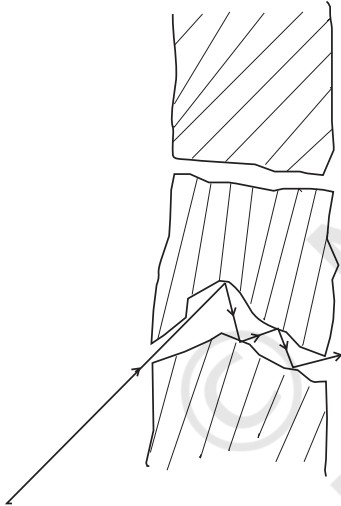
चित्र 12.5 एक सरंघ दीवार से गुजरते हुए अणु।
