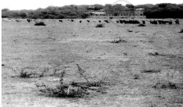
चित्र 6.4 : शुष्क मृदा
