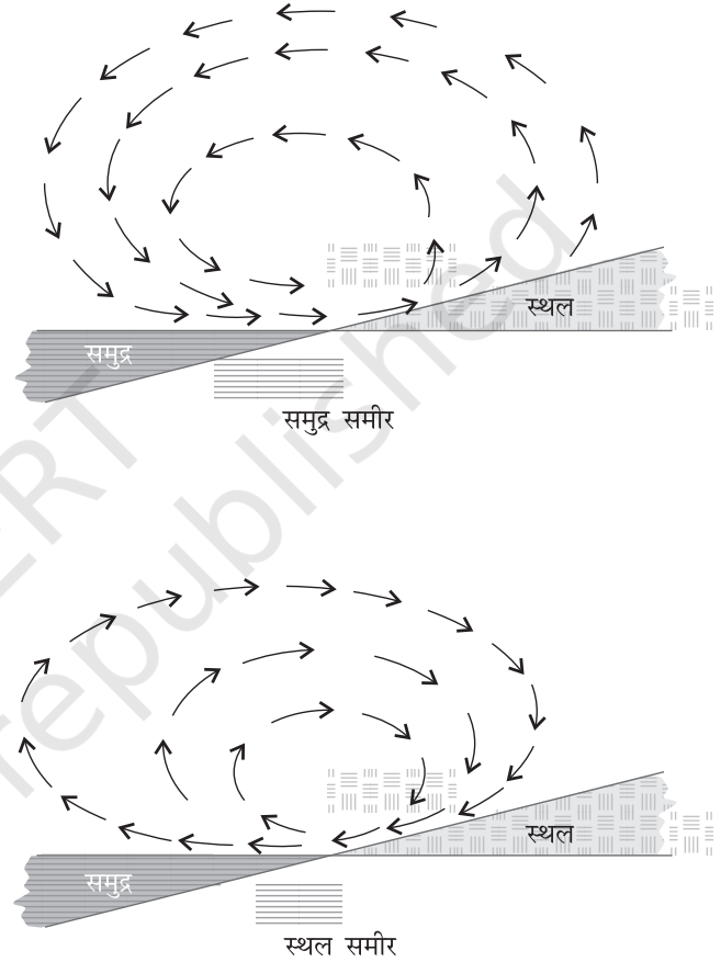
चित्र 10.7 : स्थल समीर तथा समुद्र समीर
