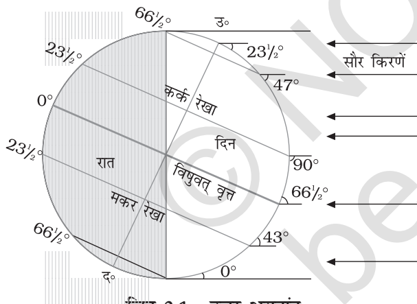
चित्र 9.1 : उत्तर अयनांत
