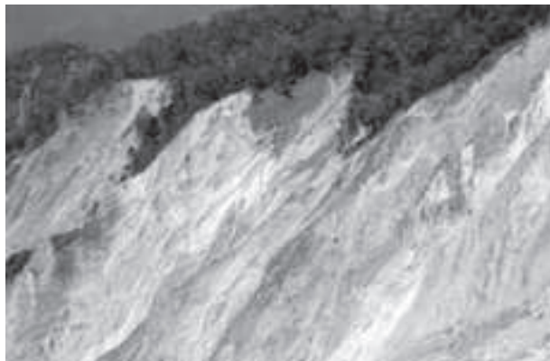
चित्र 6.7 : भारत-नेपाल सीमा, उत्तर प्रदेश में शारदा नदी के निकट शिवालिक हिमालय शृंखलाओं में भूस्खलन स्कार
