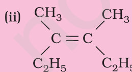
समपक्ष-3, 4-डाइमेथिल हेक्स-3-ईन
