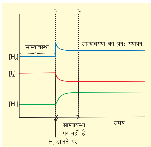
चित्र 7.8 \text{H}_2(\text{g}) + \text{I}_2(\text{g}) \rightleftharpoons 2\text{HI}(\text{g}) अभिक्रिया में साम्यावस्था पर \text{H}_2 के डालने पर अधिकारकों एवं उत्पादों के सांद्रण में परिवर्तन
